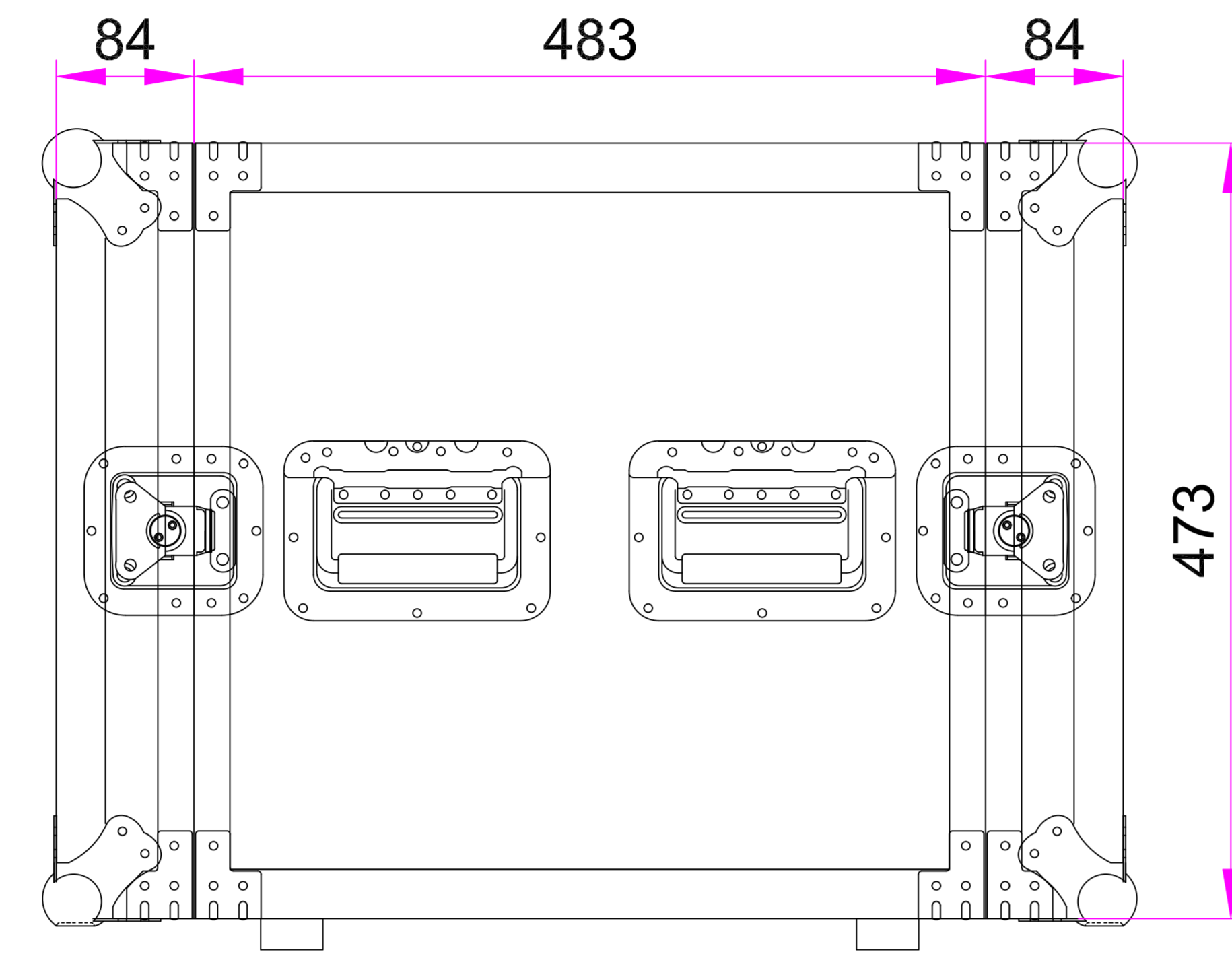
前后视图
