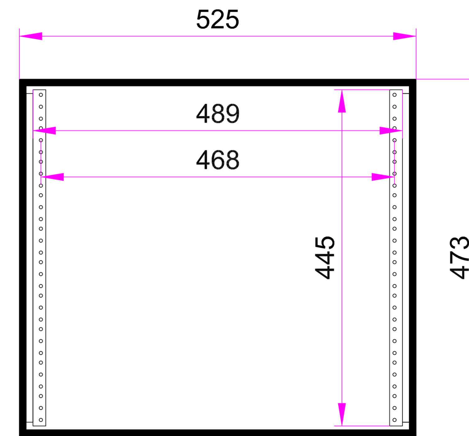
内视图
