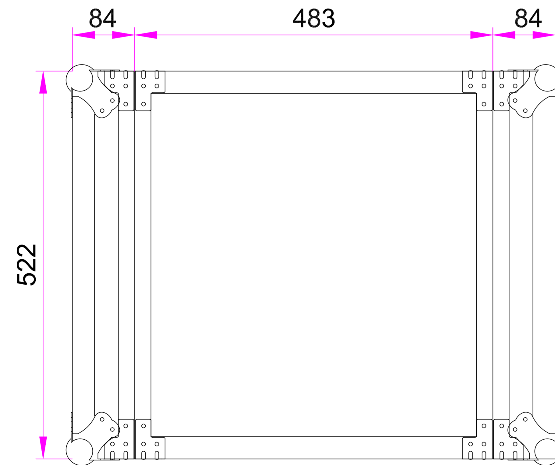
俯视图
