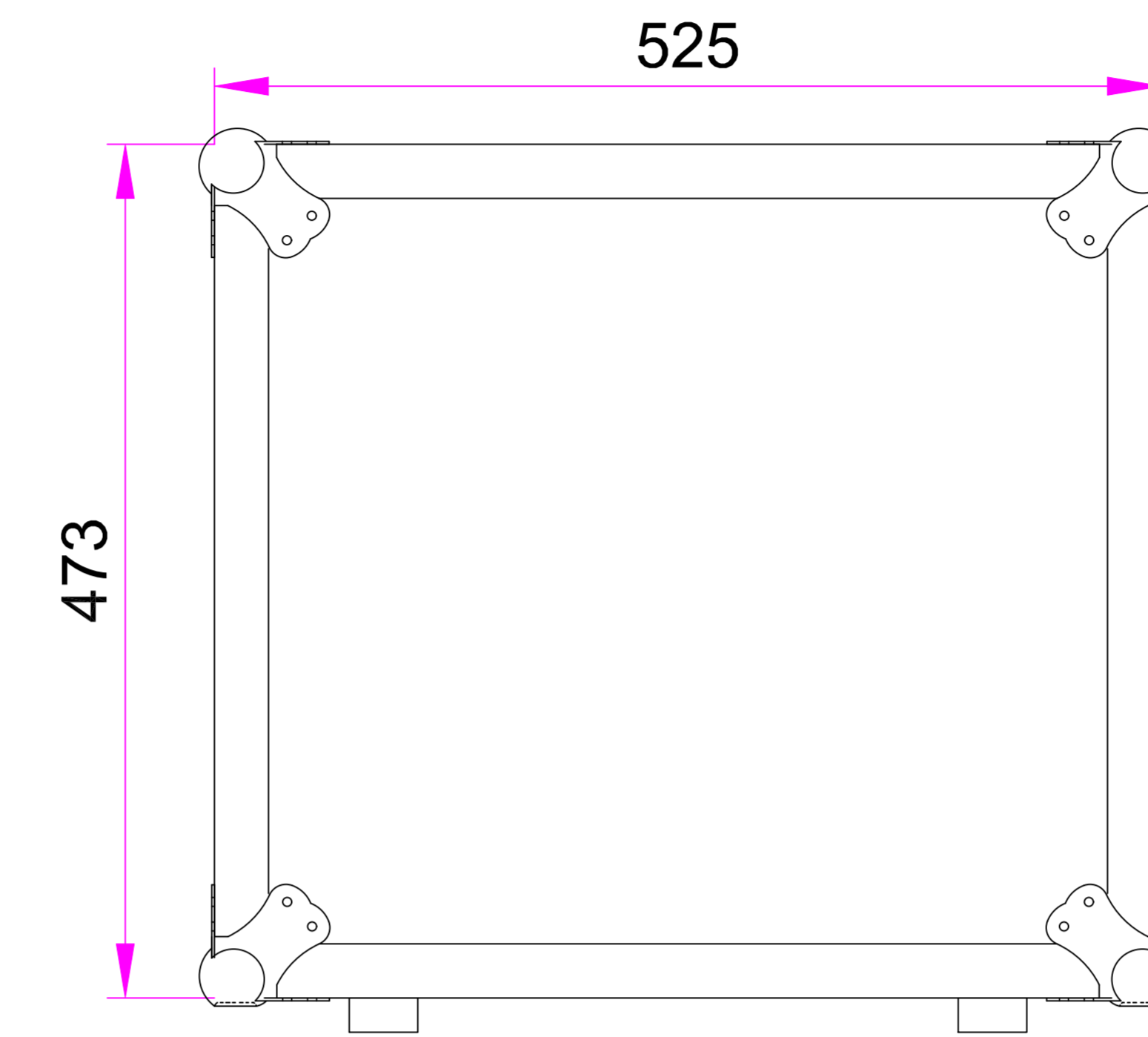
左右视图
