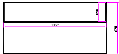
D-D视图
