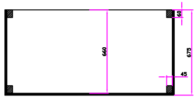
C-C视图
