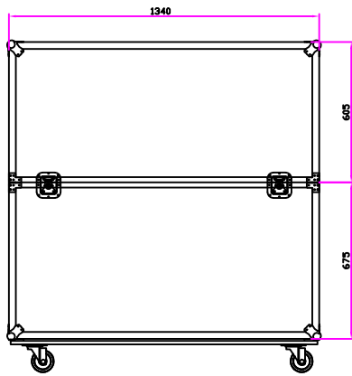
前后视图
